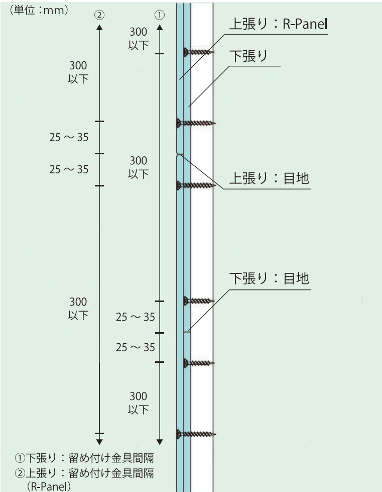
内壁：鉛直方向断面
