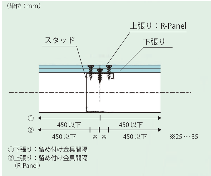
内壁：水平方向断面
